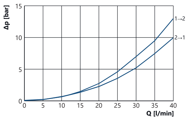
Charakterystyka strat ciśnienia ( \Delta p/Q ) MSVT-22
