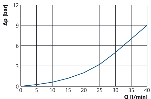
Charakterystyka strat ciśnienia ( \Delta p/Q ) MSVT-07
